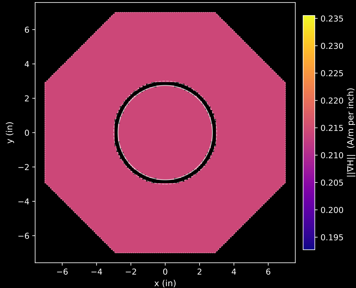
Gradient magnitude
